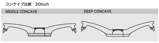
マットブラック (MBL) (ディープコンケイブ) STEP RIM 21, コンボジットハブブラッシュド (P8U) (ミドルコンケイブ) STEP RIM 21, ブラッシュド (BRU) (ミドルコンケイブ) 20, マットシルバー (MSL) (ディープコンケイブ) 20, ハブフィニッシュ (PP2) (ディープコンケイブ) 20
